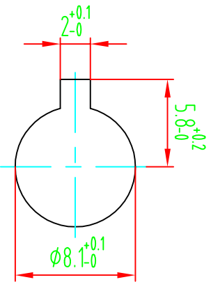
面板开孔尺寸
